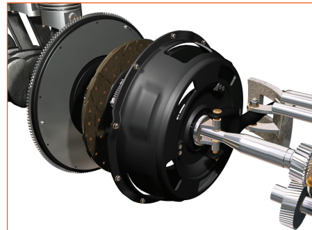
2 CLUTCH
