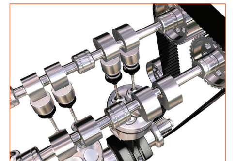
2 CAMSHAFT
